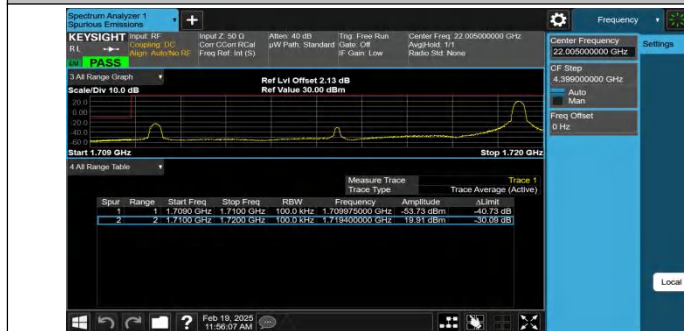
Band4-10MHz-QPSK-20000-1RB#49-PASS
