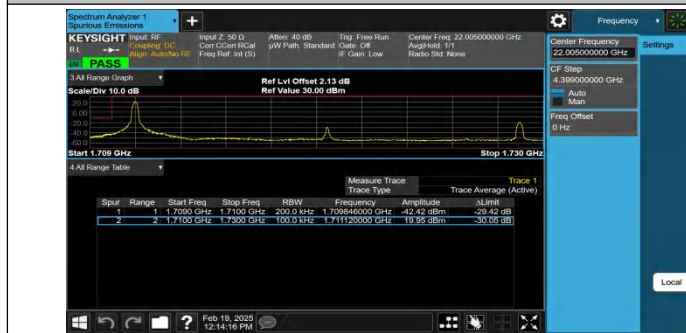
Band4-20MHz-QPSK-20050-1RB#0-PASS
