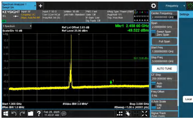
Band2-20MHz-QPSK-18900-1RB#99-1000~3000-PASS
