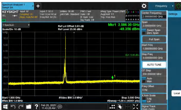
Band2-20MHz-QPSK-18700-1RB#99-1000~3000-PASS
