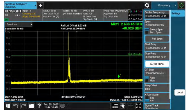
Band2-20MHz-QPSK-18900-1RB#0-1000~3000-PASS
