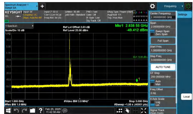
Band2-20MHz-QPSK-18700-1RB#0-1000~3000-PASS
