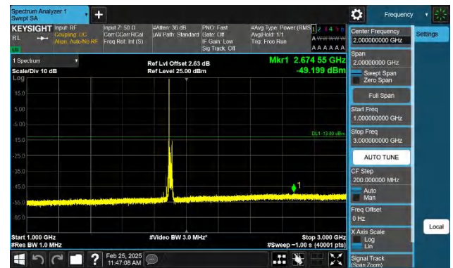
Band2-20MHz-QPSK-19100-1RB#0-1000~3000-PASS
