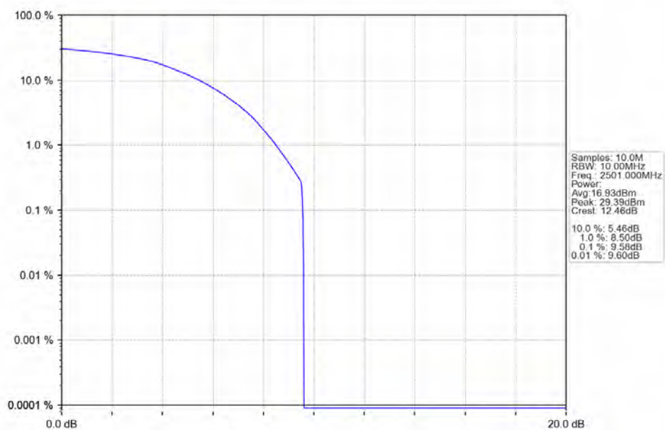
Band41_10MHz_256QAM_LCH_2501MHz_RB_50_0_NTNV
