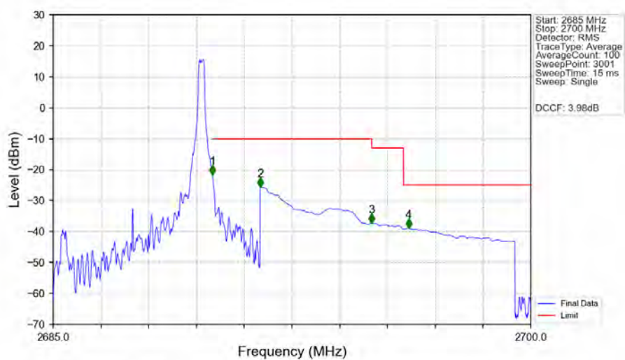
Band41_5MHz_QPSK_HCH_2687.5MHz_RB_1_24_NTNV
