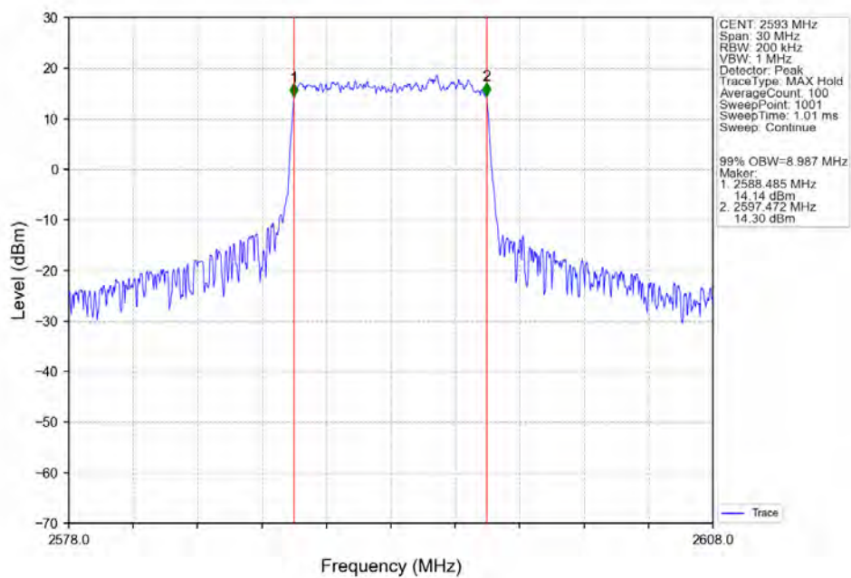
Band41_10MHz_64QAM_MCH_2593MHz_RB_50_0_NTNV
