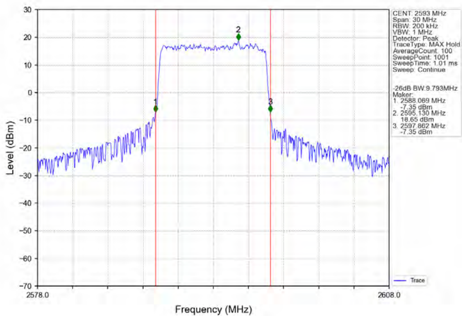
Band41_10MHz_64QAM_MCH_2593MHz_RB_50_0_NTNV
