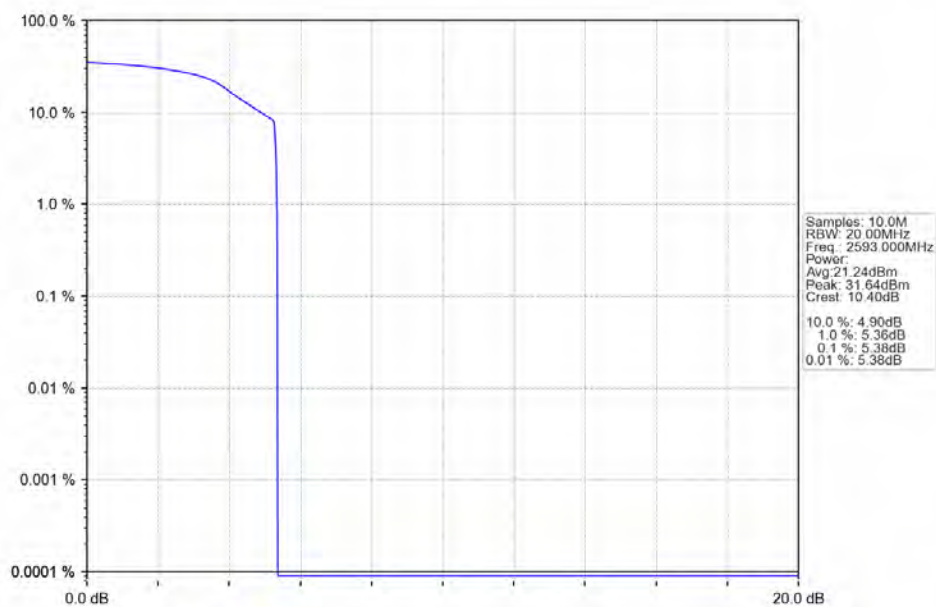
Band41_15MHz_QPSK_MCH_2593MHz_RB_75_0_NTNV
