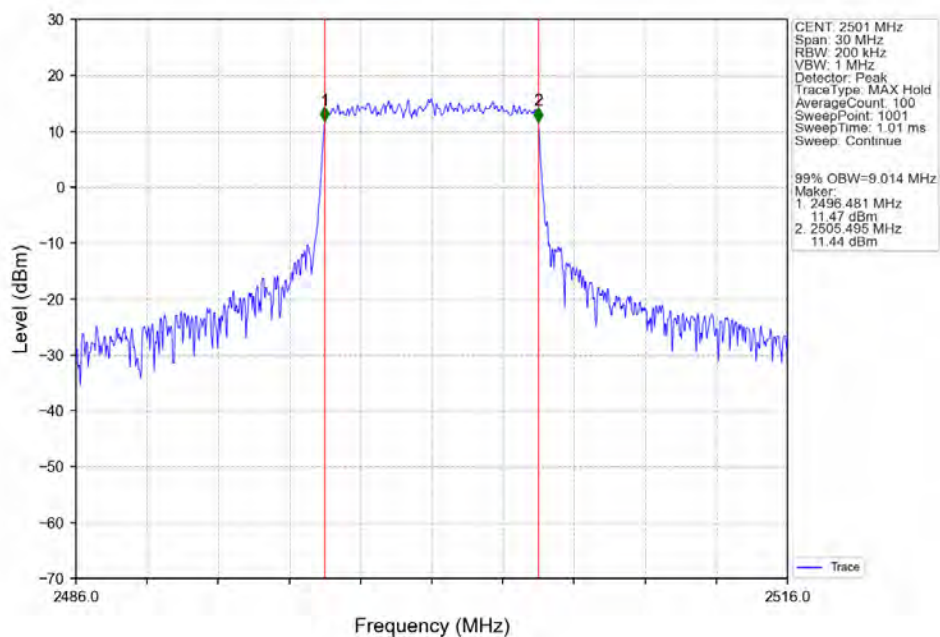
Band41_10MHz_256QAM_LCH_2501MHz_RB_50_0_NTNV
