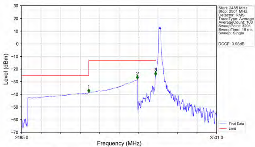
Band41_5MHz_QPSK_LCH_2498.5MHz_RB_1_0_NTNV
