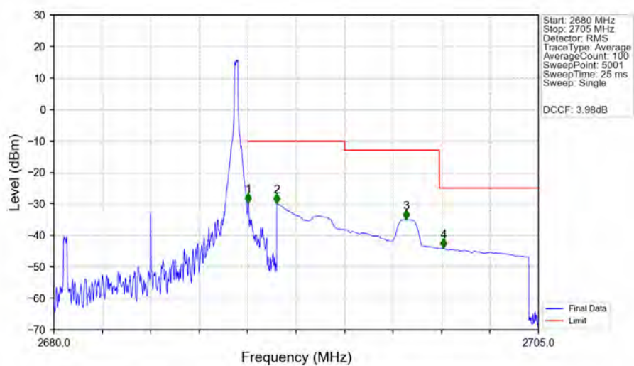
Band41_10MHz_QPSK_HCH_2685MHz_RB_1_49_NTNV
