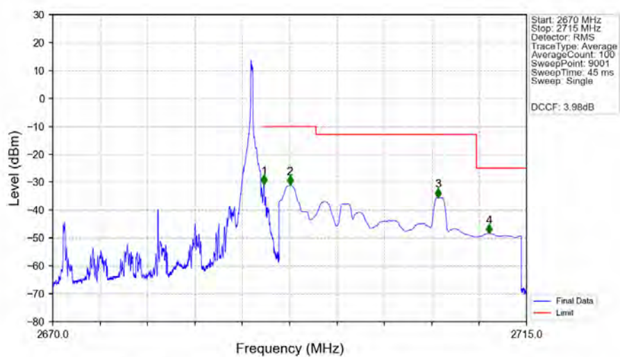
Band41_20MHz_QPSK_HCH_2680MHz_RB_1_99_NTNV
