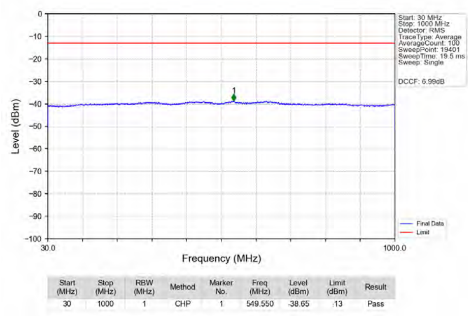
n78e 30kHz SISO NTN 60MHz CP-OFDM QPSK 3480MHz Edge 1RB Left Ant1
