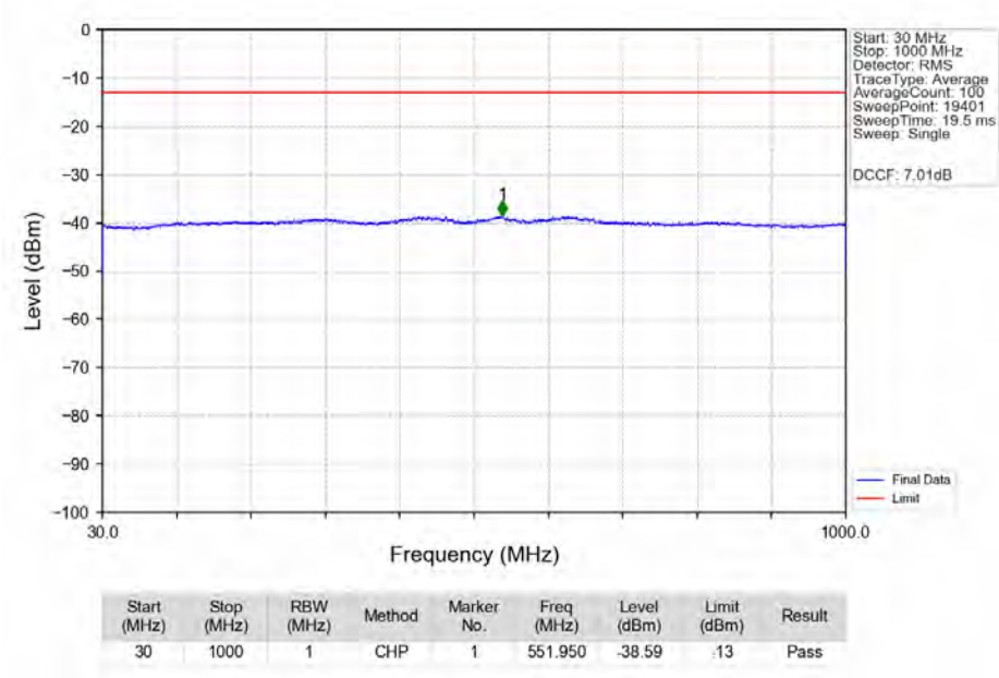
n78e 30kHz SISO NTN 90MHz CP-OFDM QPSK 3500.01MHz Edge 1RB Left Ant1
