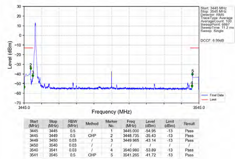
n78e 30kHz SISO NTN 90MHz CP-OFDM QPSK 3495MHz Inner 1RB Left Ant1
