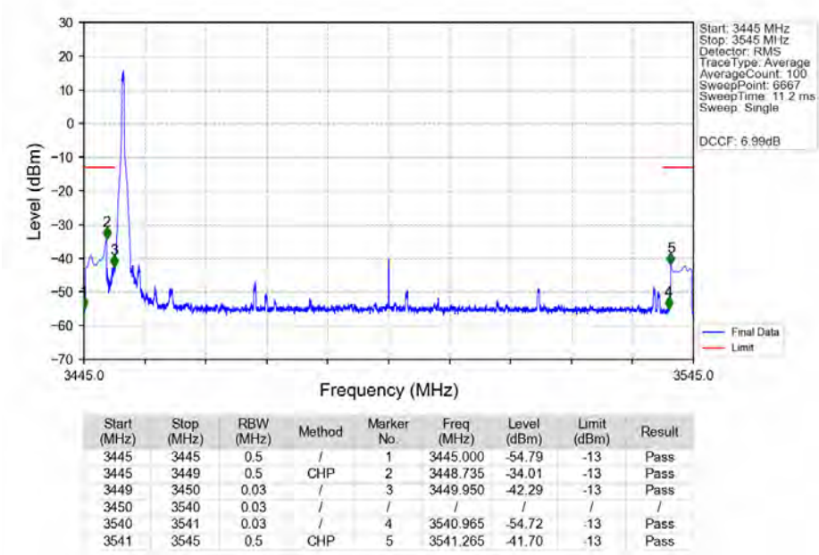
n78e_30kHz_SISO_NTNV_90MHz_DFT-s-OFDM_PI/2_BPSK_3495MHz_Inner_1RB_Left_Ant1
