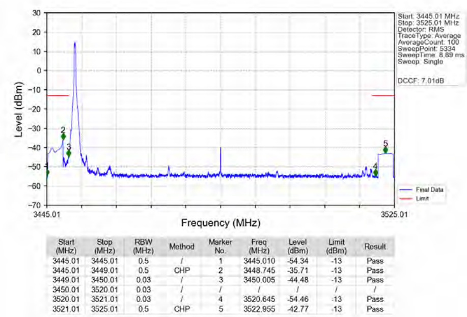
n78e 30kHz SISO NTN 70MHz CP-OFDM QPSK 3485.01MHz Inner 1RB Left Ant1
