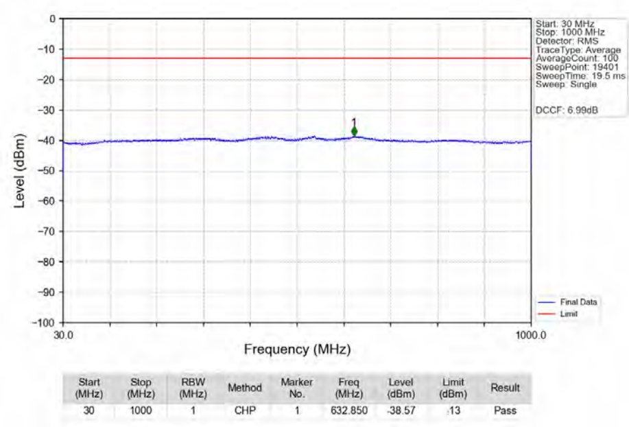
n78e 30kHz SISO NTN 70MHz CP-OFDM QPSK 3500.01MHz Edge 1RB Left Ant1
