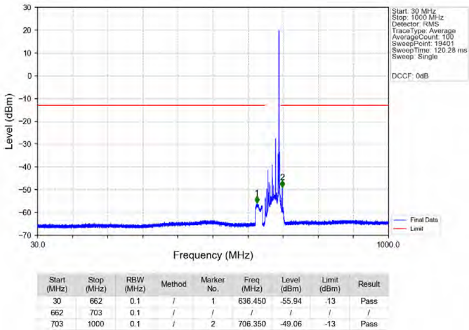
n71 15kHz SISO NTN 20MHz CP-OFDM QPSK 688MHz Edge 1RB Right Ant1
