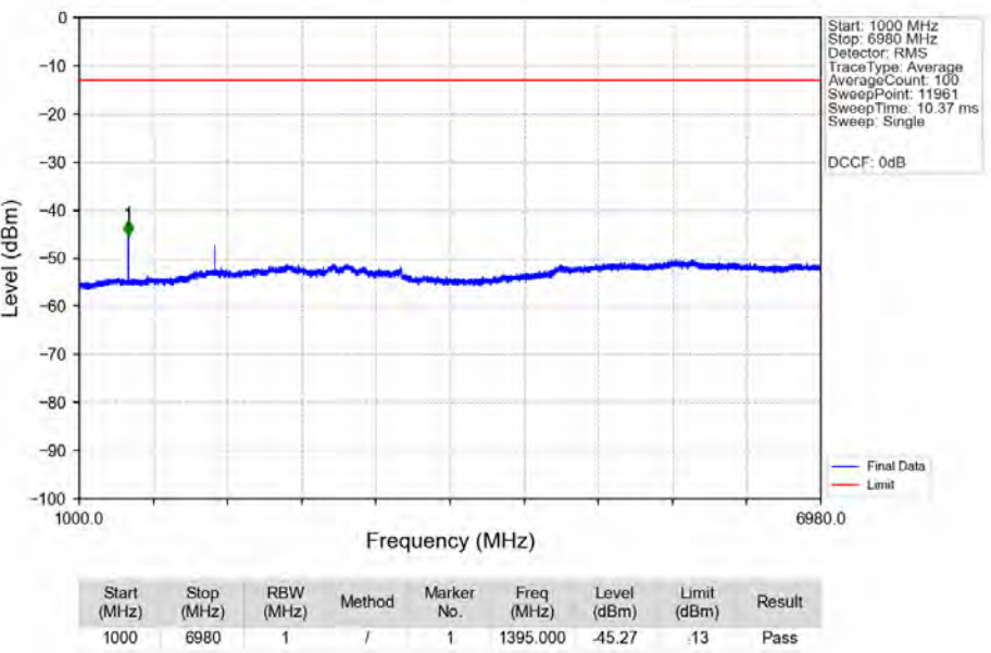
n71 15kHz SISO NTN 20MHz CP-OFDM QPSK 688MHz Edge 1RB Right Ant1
