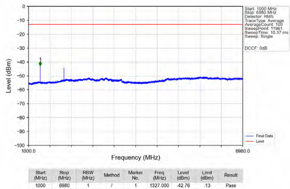
n71 15kHz SISO NTN 15MHz DFT-s-OFDM QPSK 670.5MHz Edge 1RB Left Ant1
