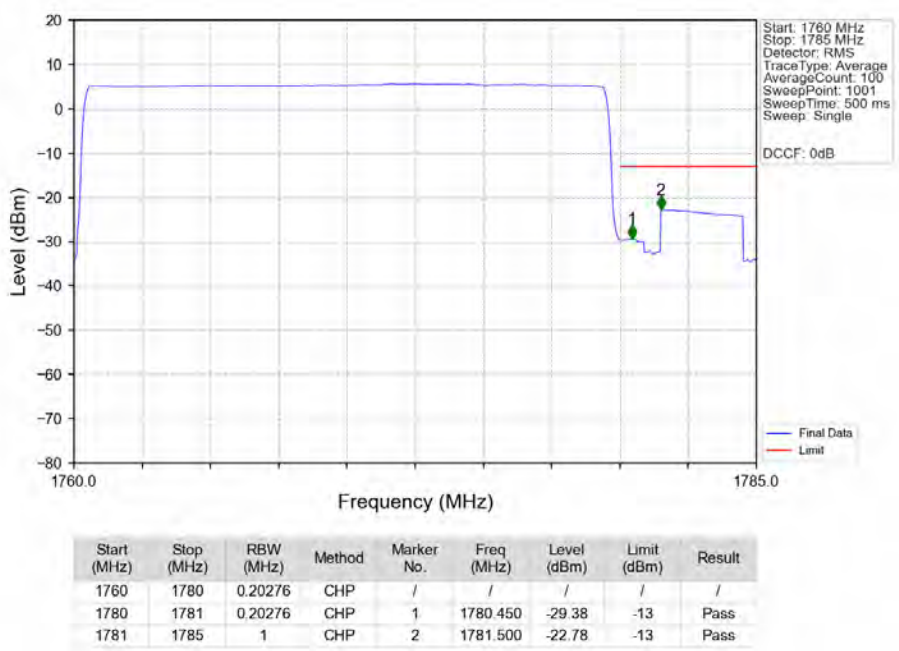
n66 15kHz SISO NTN 20MHz CP-OFDM QPSK 1770MHz Inner 1RB Right Ant1
