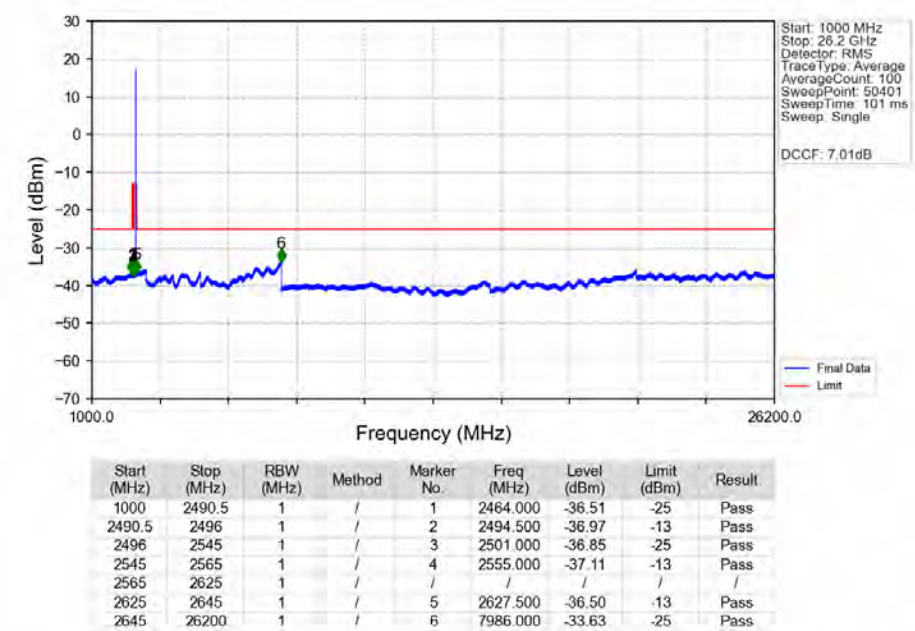
n38 30kHz MIMO NTN 25MHz CP-OFDM QPSK 2607.5MHz Edge 1RB Right Ant1
