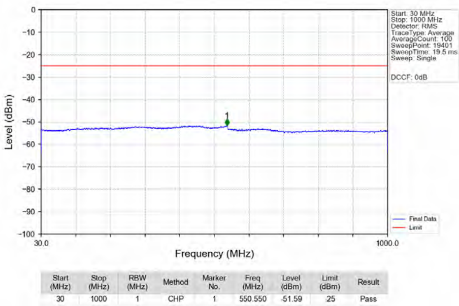
n7 15kHz SISO NTN 50MHz DFT-s-OFDM QPSK 2535MHz Edge 1RB Left Ant1
