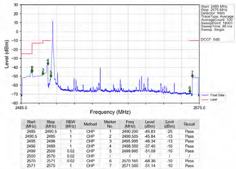
n7 15kHz SISO NTN 50MHz DFT-s-OFDM QPSK 2535MHz Edge 1RB Left Ant1
