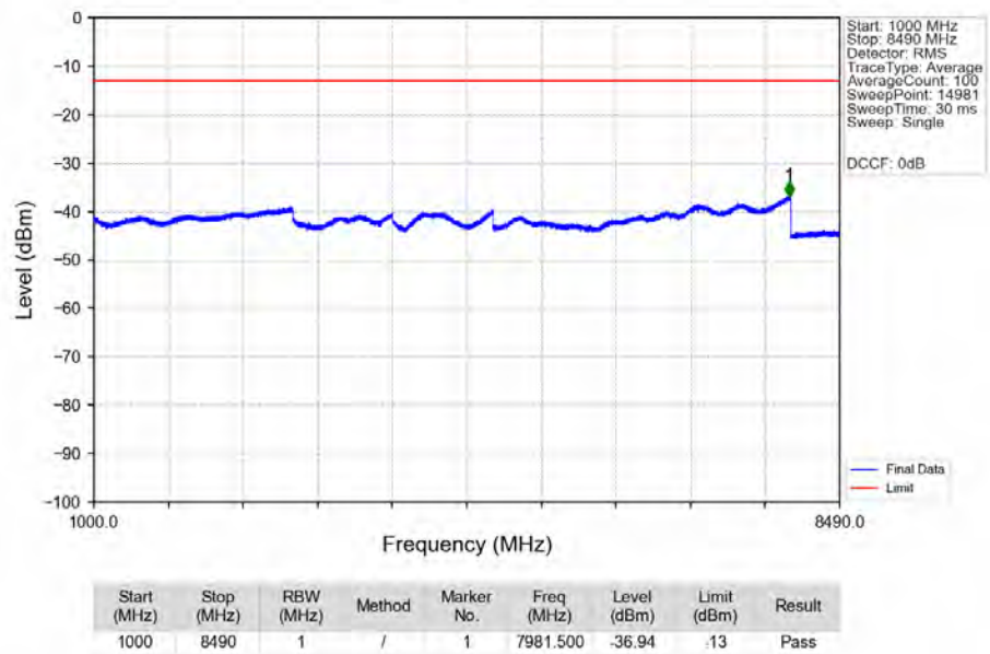
n5 15kHz MIMO NTN 20MHz CP-OFDM QPSK 839MHz Edge 1RB Right Ant2
