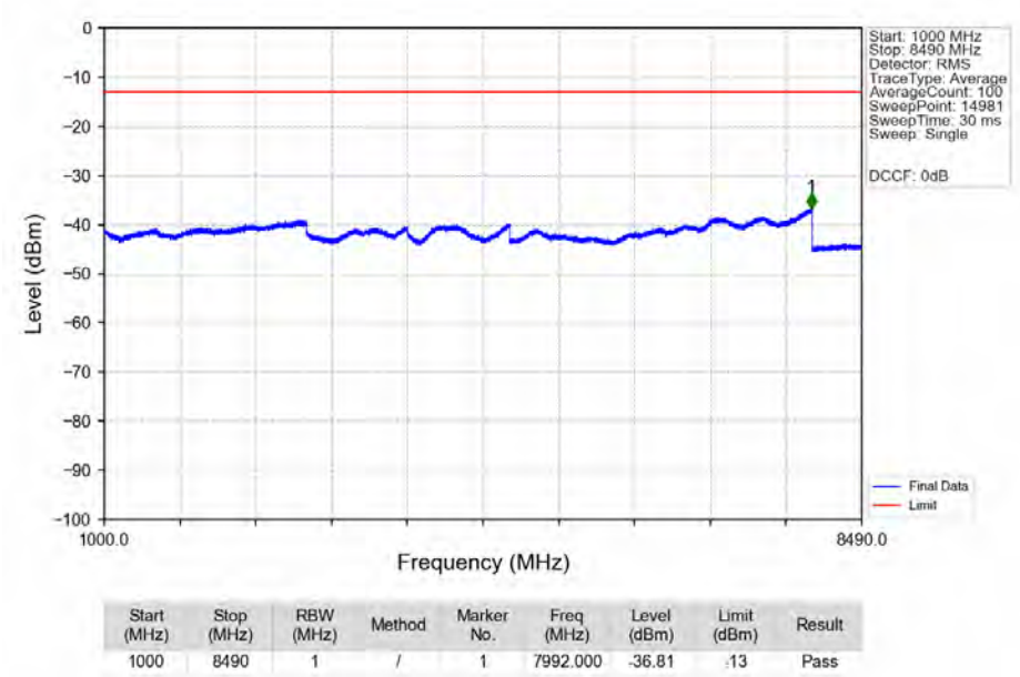
n5 15kHz MIMO NTN 20MHz CP-OFDM QPSK 834MHz Edge 1RB Left Ant2
