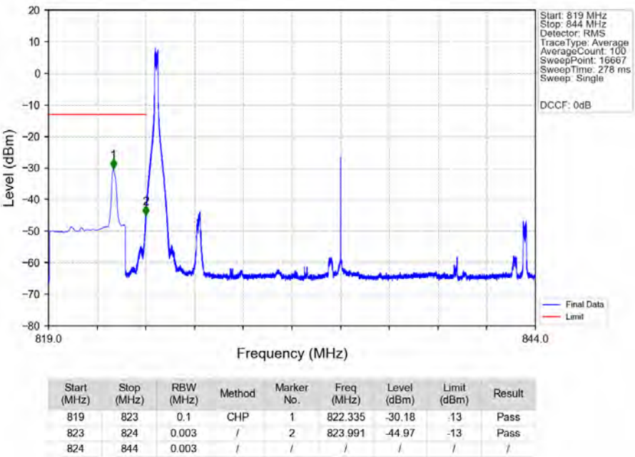
n5 15kHz MIMO NTNv 20MHz CP-OFDM QPSK 834MHz Edge 1RB Left MIMO
