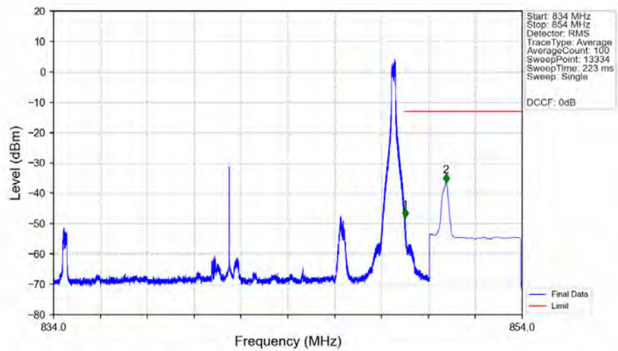
n5 15kHz MIMO NTNV 15MHz CP-OFDM QPSK 841.5MHz Edge 1RB Right Ant1
