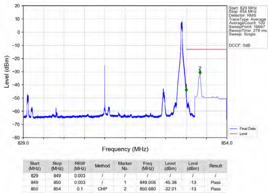
n5 15kHz MIMO NTN 20MHz CP-OFDM QPSK 839MHz Edge 1RB Right MIMO
