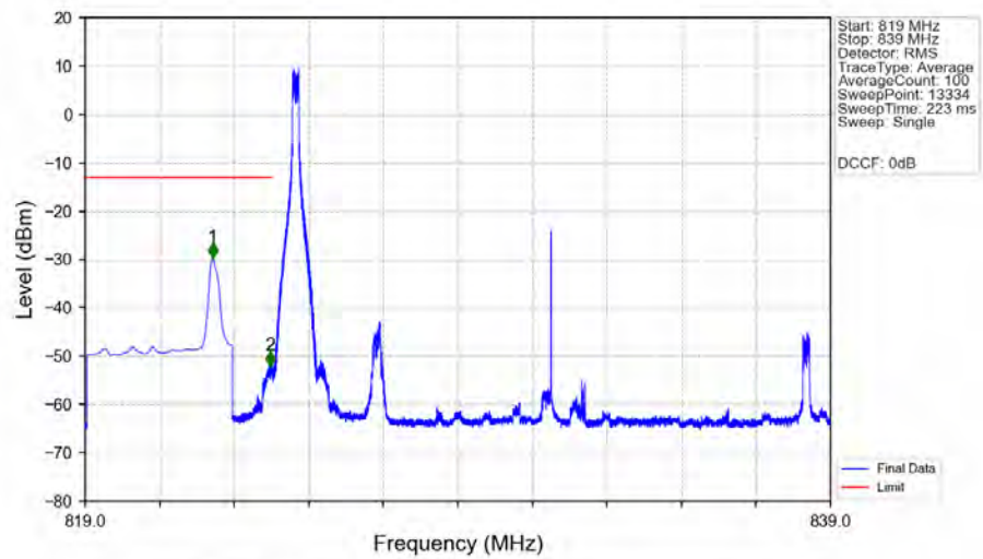
n5 15kHz MIMO NTNV 15MHz CP-OFDM QPSK 831.5MHz Inner 1RB Left MIMO
