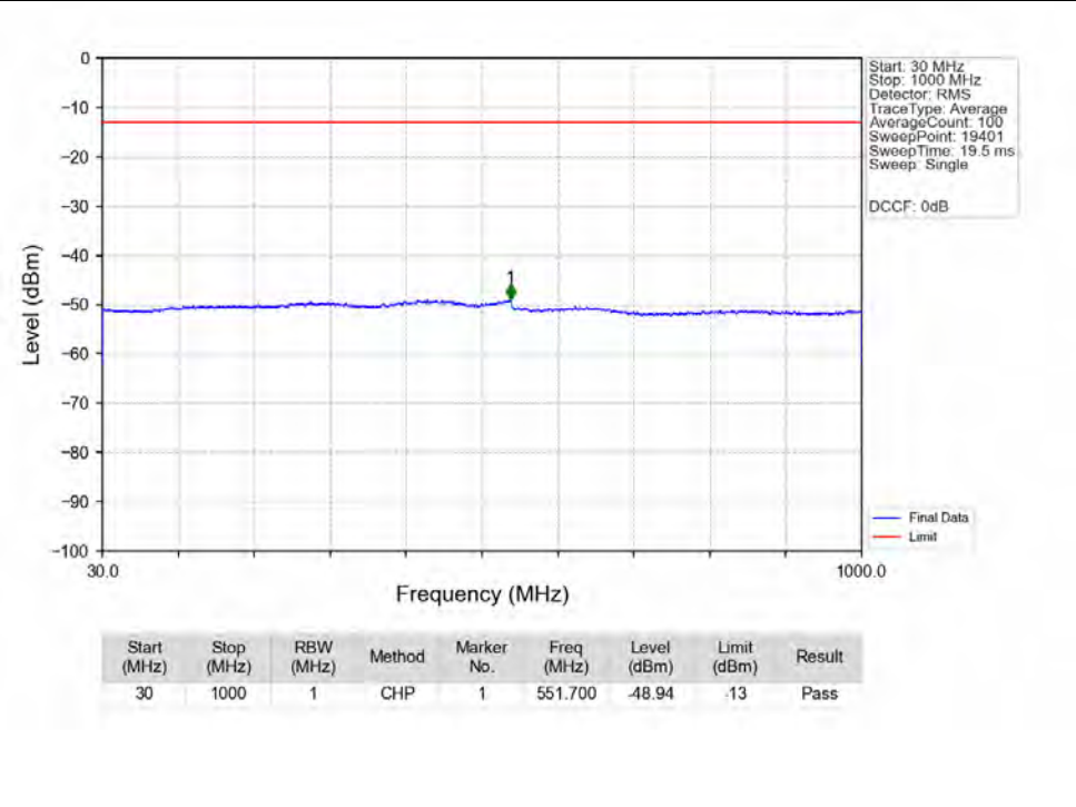
n2 15kHz MIMO NTN 10MHz DFT-s-OFDM QPSK 1905MHz Edge 1RB Right Ant2
