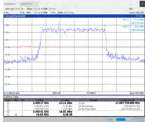
1-N78-3450-3550-PC2-30-20-M-4-DFT-64QAM-Out r_Full-50@0-Ant0-17.898-19.040-≤20-PASS
