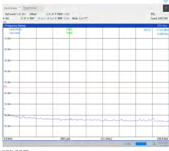
1-N41-30-100-M-1-DFT-PI2BPSK-Inner_1RB_Left-1 @1-0.009-0.15-Ant0-0.01--77.69--55-PASS
