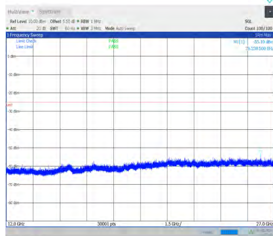
1-N41-30-100-L-1-DFT-PI2BPSK-Inner_1RB_Left-1 @1-12000-27000-Ant0-26238.50--55.10--25-PASS
