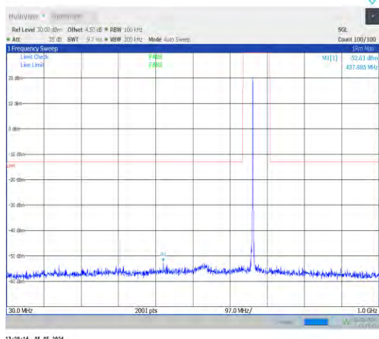
1-N71-PC3-15-20-M-1-DFT-PI2BPSK-Inner_1RB_L eft-1@1-30-1000-Ant0-437.89--52.61--13-PASS
