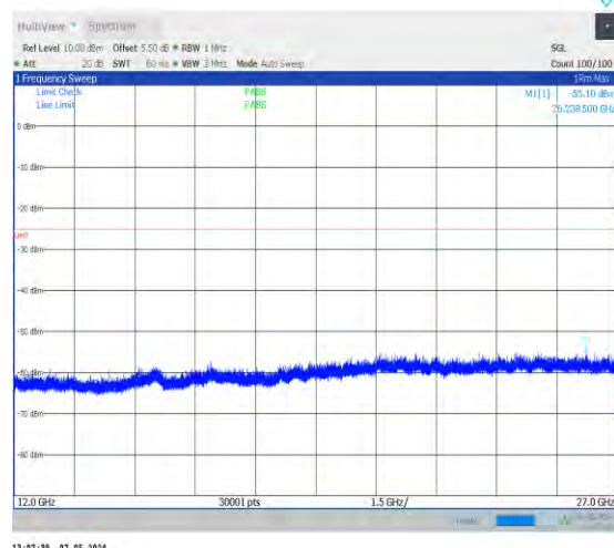
1-N41-30-100-L-1-DFT-PI2BPSK-Inner_1RB_Left-1 @1-12000-27000-Ant0-26238.50--55.10--25-PASS
