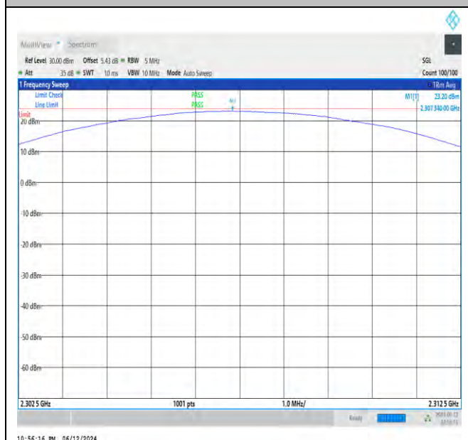
NTVN_N30_PC3_15_5_L_TID6_NS_01_2302.5_2312.5_ #1
