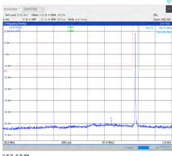
1-N14-PC3-15-10-H-1-DFT-PI2BPSK-Inner_1RB_L eft-1@1-30-1000-Ant0-650.80--58.72--13-PASS
