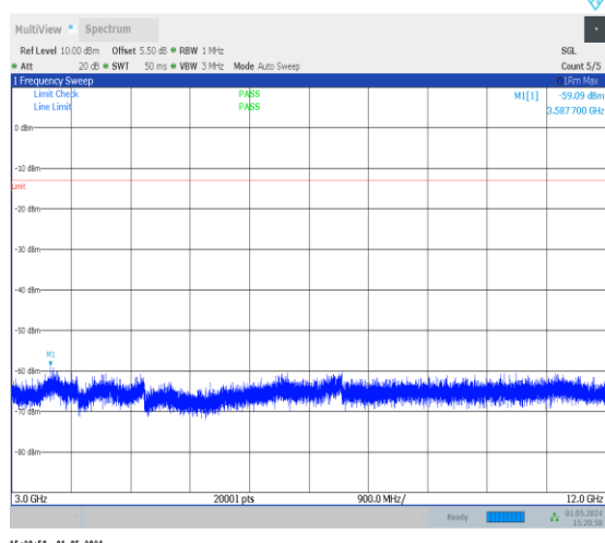
1-N13-PC3-15-10-M-1-DFT-PI2BPSK-Inner_1RB_L eft-1@1-3000-12000-Ant0-3587.70--59.09--13-PAS S
