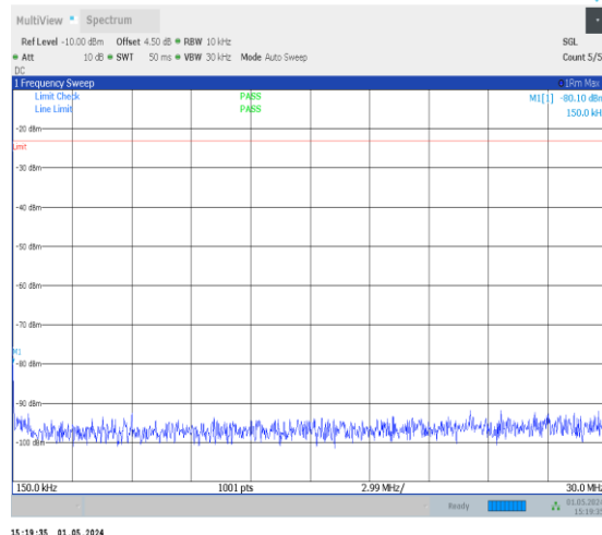
1-N13-PC3-15-10-L-1-DFT-PI2BPSK-Inner_1RB_Left -1@1-0.15-30-Ant0-0.15--80.10--23-PASS
