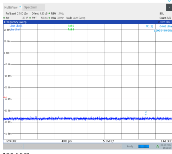
1-N13-PC3-15-10-M-1-DFT-PI2BPSK-Inner_1RB_L eft-1@1-1559-1610-Ant0-1602.04--54.68--40-PASS
