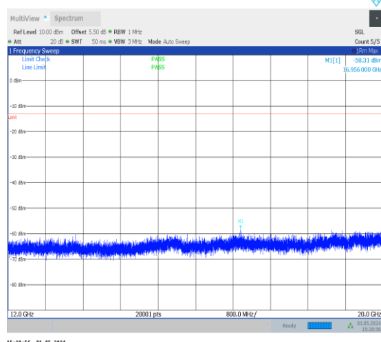
1-N13-PC3-15-10-M-1-DFT-PI2BPSK-Inner_1RB_L ef t-1@1-12000-20000-Ant0-16956.00--58.31--13-PASS
