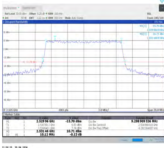
1-N7-PC3-15-10-M-6-CP-QPSK-Outer_Full-52@0-Ant0-9.299-10.120-≤10-PASS
