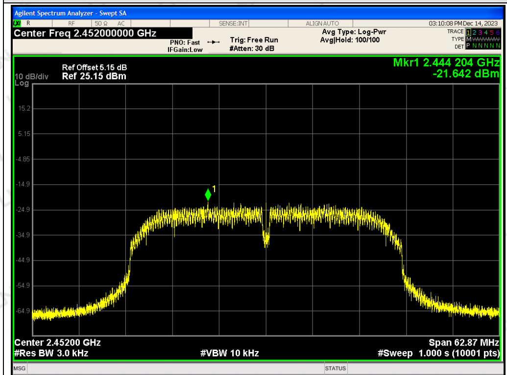
CH09: 2452MHz
