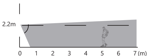
Vista dall'alto
