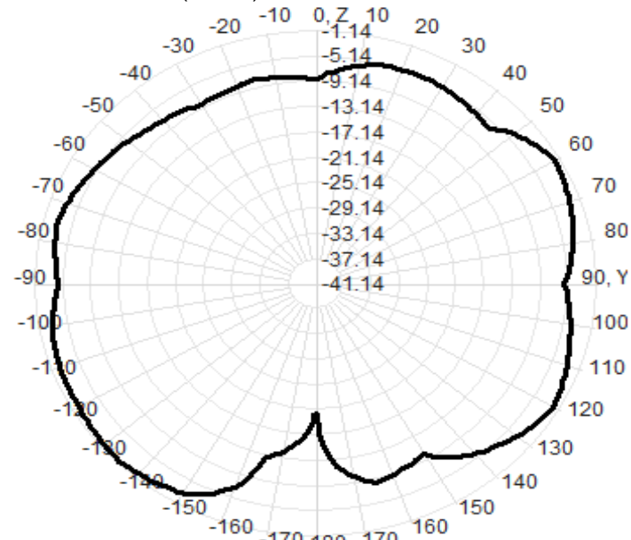
2490.0MHz Total(E2-YZ), Max=-1.65dBi
