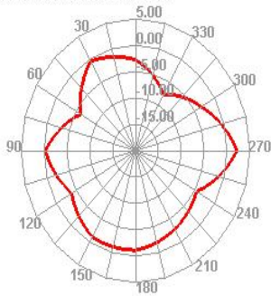
2450.000MHz E1
