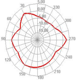
2500.000MHz E1
