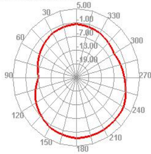
2400.000MHz H
