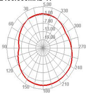
2450.000MHz H
