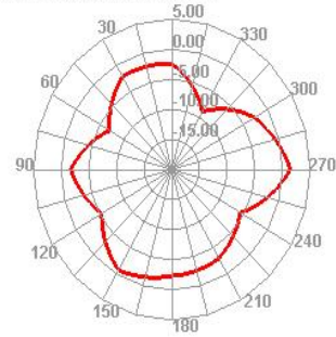
2400.000MHz E1
