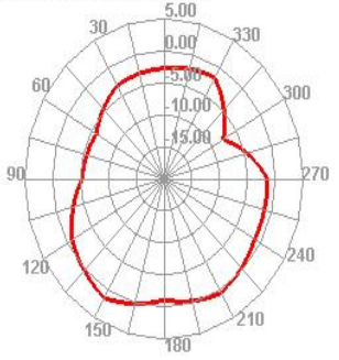
2450.000MHz E2
