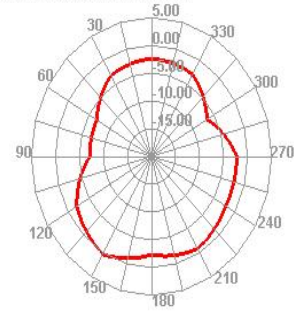
2400.000MHz E2
