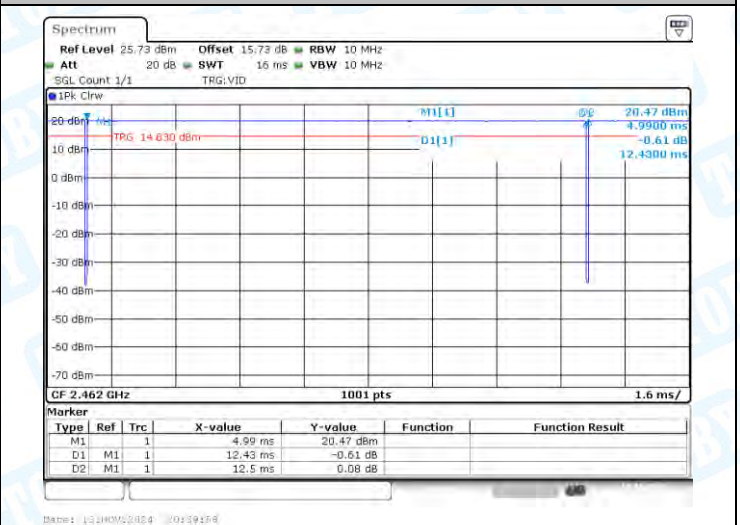
NTVN-11B-CDD-Ant2-2462
