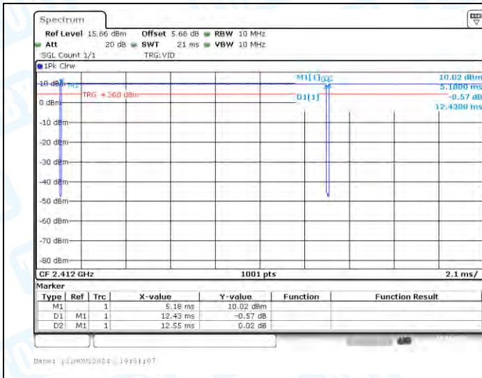
NTVN-11B-CDD-Ant1-2412
