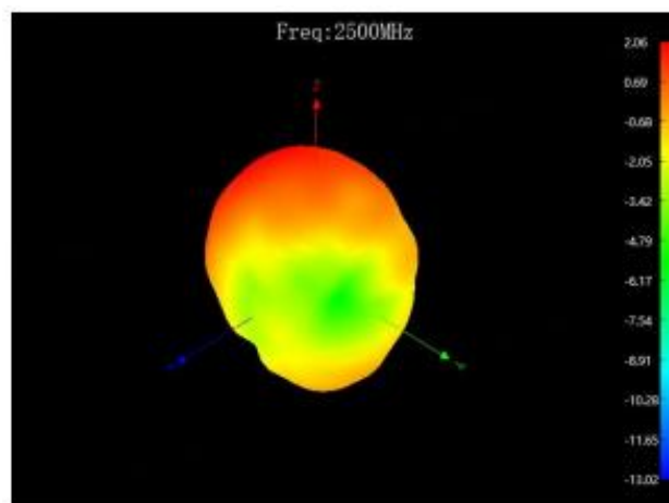
2500MHz 3D
