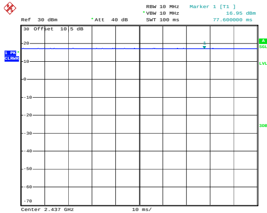
b_2437MHz_Chain 0
