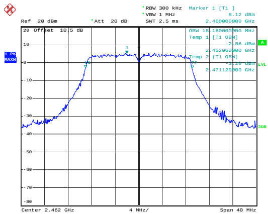
n20_2462MHz_Chain 0
