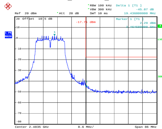
n20_2462MHz_Chain 0
