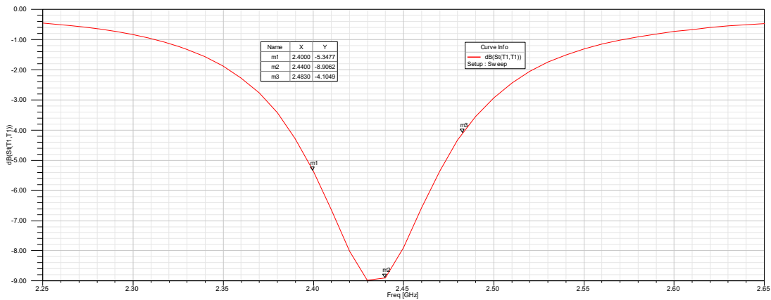
1-2 PIFA C Type antenna S11 Parameter diagram
