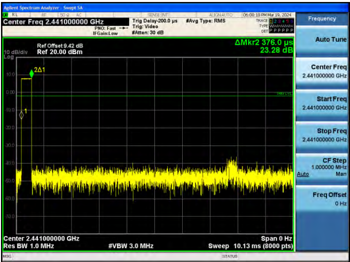
DH1_Ant1_Hop
