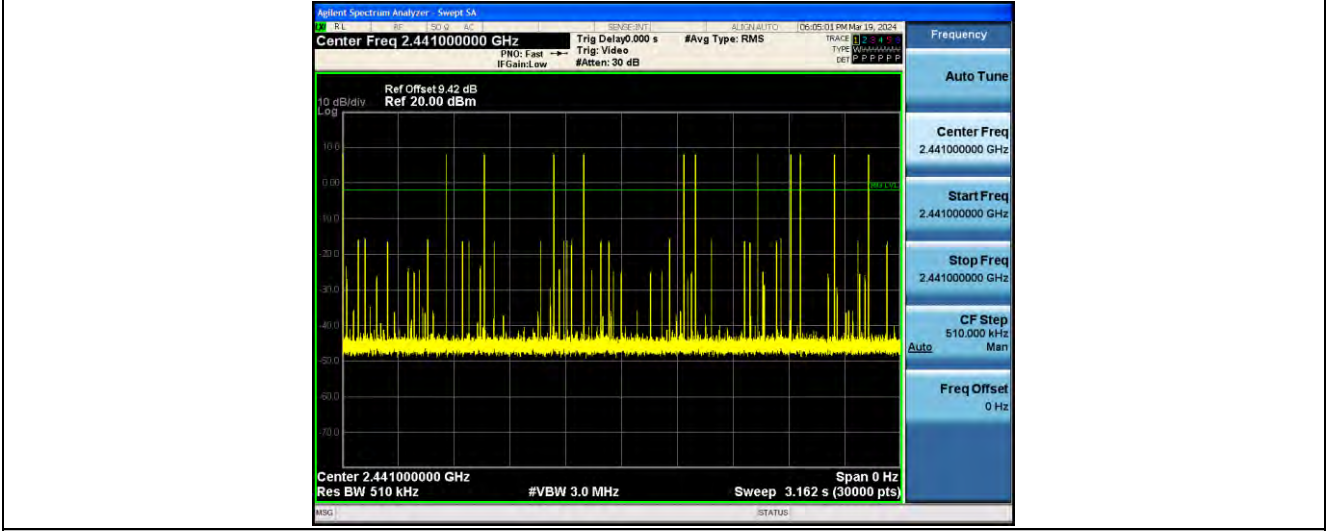
2DH1_Ant1_Hop
