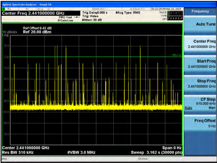
3DH1_Ant1_Hop
