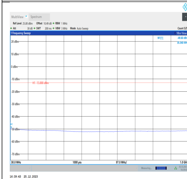
Band2-20MHz-QPSK-19100-PASS
