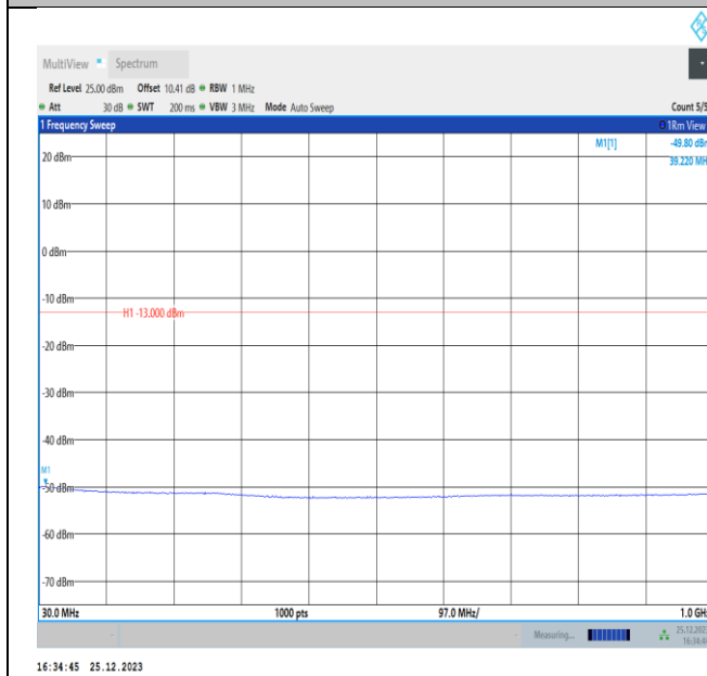
Band2-20MHz-QPSK-18700-PASS
