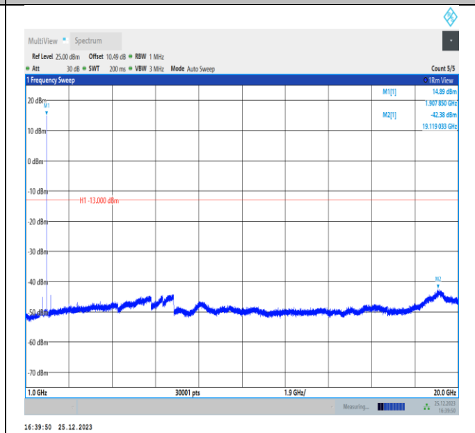
Band2-20MHz-QPSK-19100-PASS
