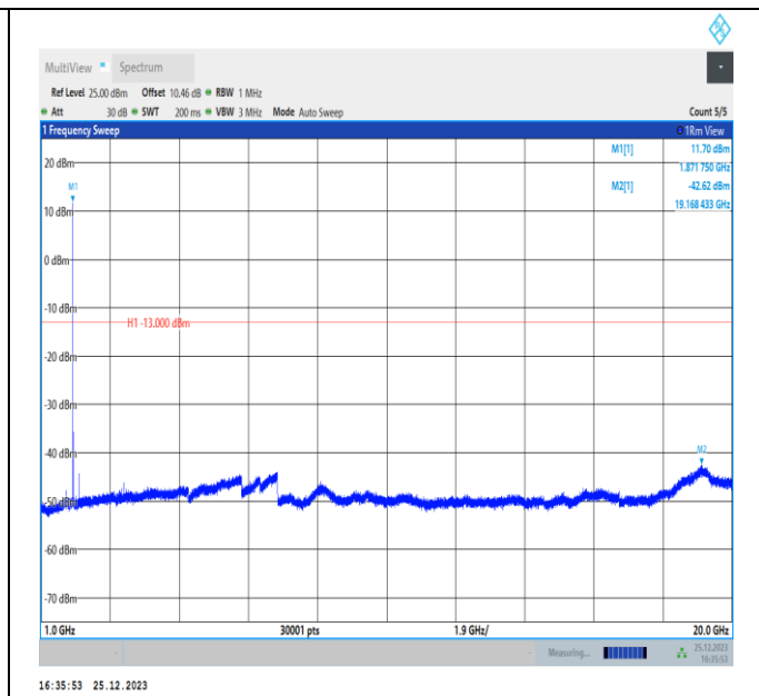
Band2-20MHz-QPSK-18900-PASS
