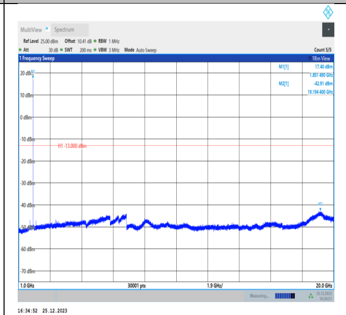
Band2-20MHz-QPSK-18700-PASS
