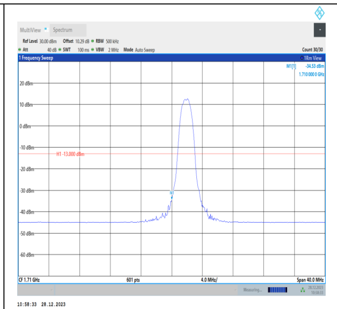
Band4-20MHz-QPSK-20050-PASS
