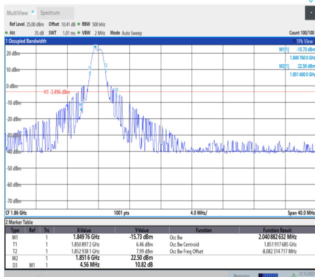
Band2-20MHz-QPSK-18700-PASS
