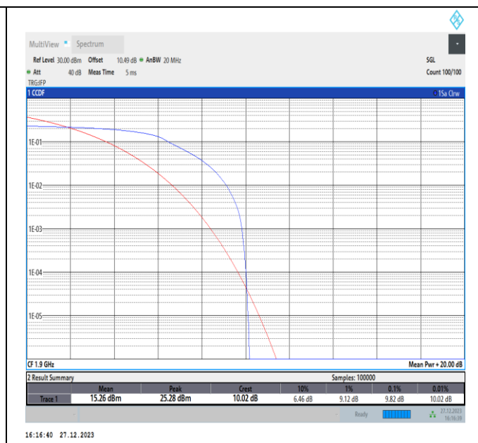
Band2-20MHz-QPSK-19100-PASS
