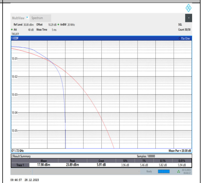
Band4-20MHz-QPSK-20050-PASS
