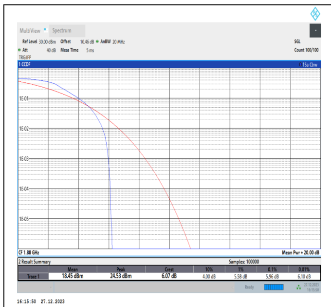
Band2-20MHz-QPSK-18900-PASS
