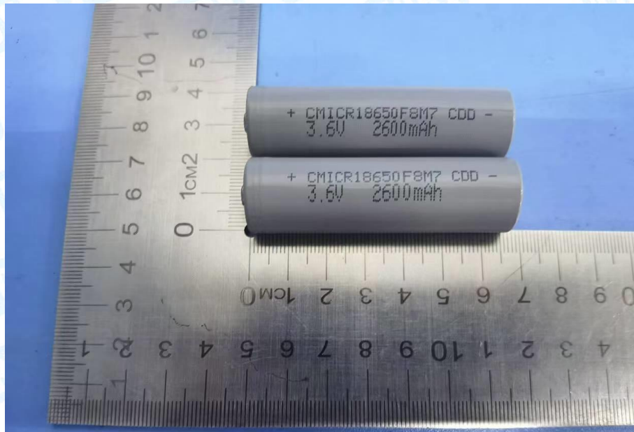
Photo 14 Battery parameters
