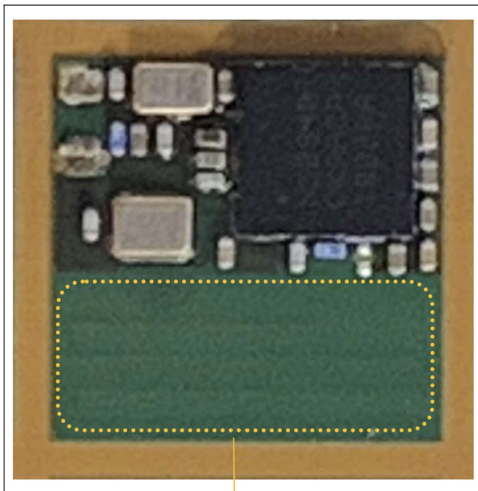
Antenna Area
