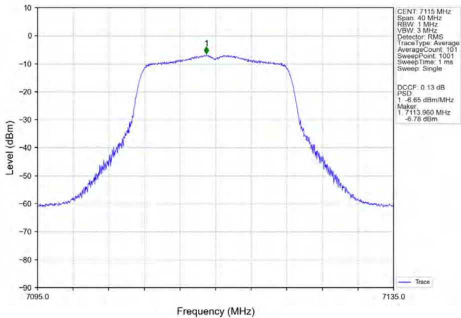
802.11a_HCH_7115MHz_Ant5_NTNV
