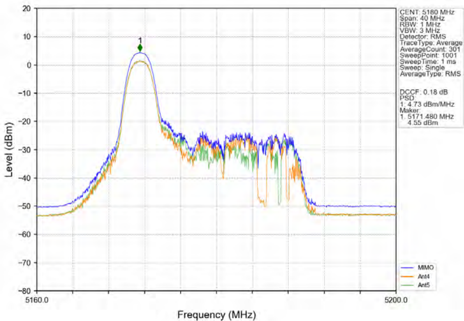
802.11ax(HEW20)_LCH_5180MHz_RU52-Ant4_NTNV
