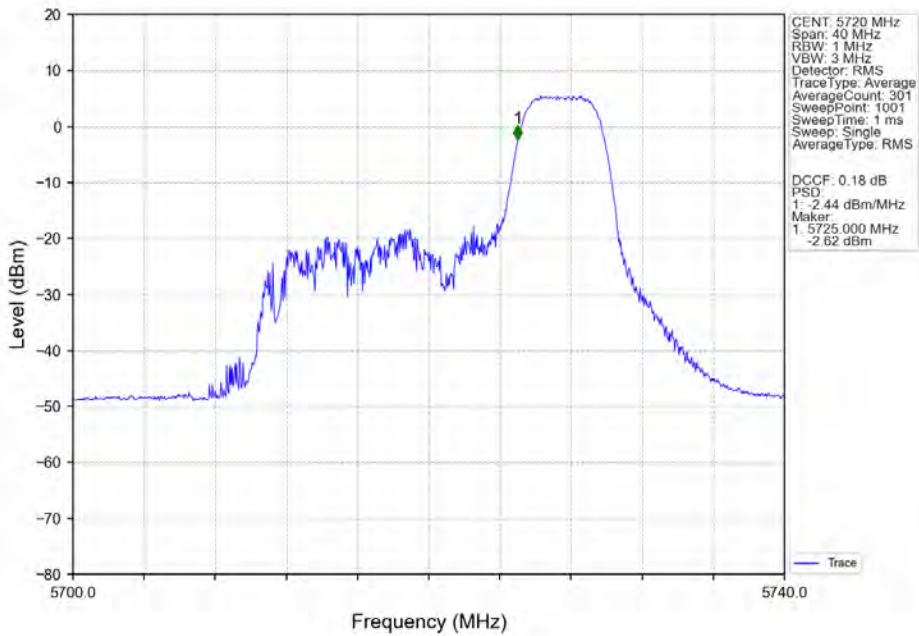
802.11ax(HEW20)_HCH_5720MHz_RU52-MIMO_NTNV
