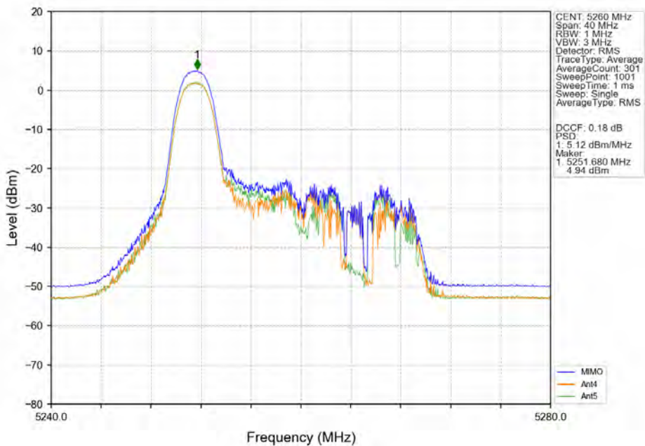
802.11ax(HEW20)_LCH_5260MHz_RU52-Ant4_NTNV
