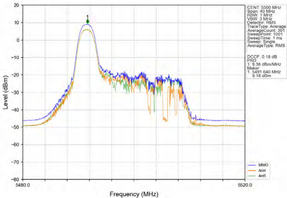
802.11ax(HEW20)_LCH_5500MHz_RU52-Ant4_NTNV
