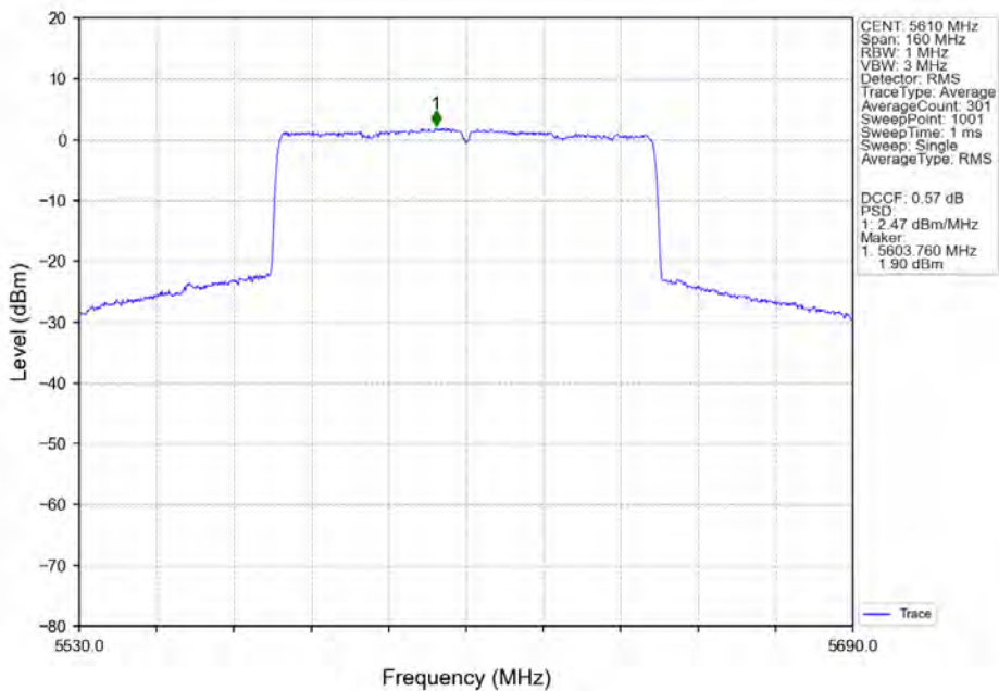
802.11ax(HEW80)_HCH_5610MHz_SU_/_MIMO_NTNV
