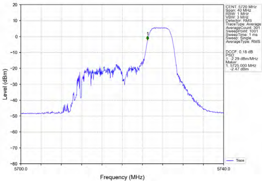
802.11ax(HEW20)_HCH_5720MHz_RU52-Ant4_NTNV
