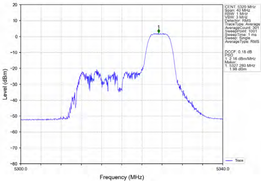
802.11ax(HEW20)_HCH_5320MHz_RU52-Ant4_NTNV
