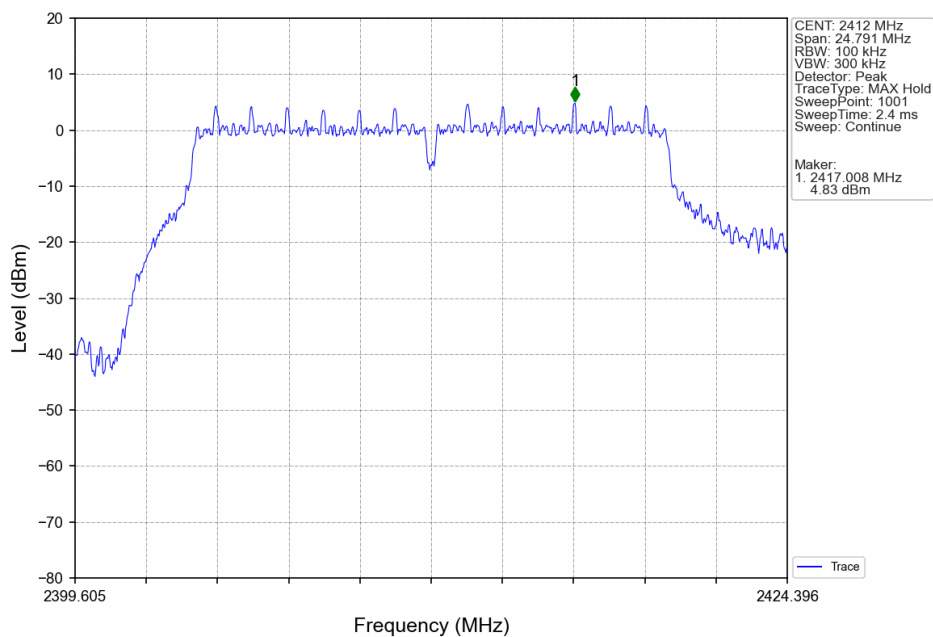
802.11g_LCH_2412MHz_Ant5 (MIMO)_NTNV
