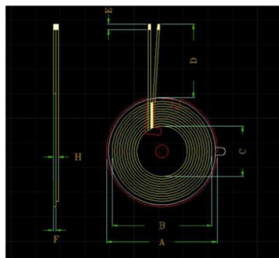
二、原理图 SCHEMATIC DIAGRAM:
