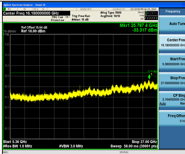
11A-Ant1-5200-5360~27000-PASS
