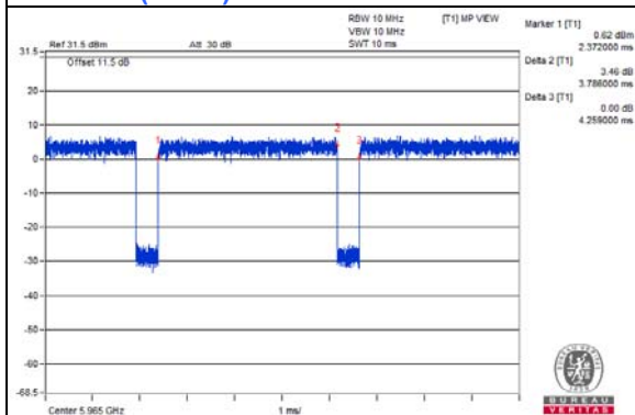
802.11ax (HE160)
