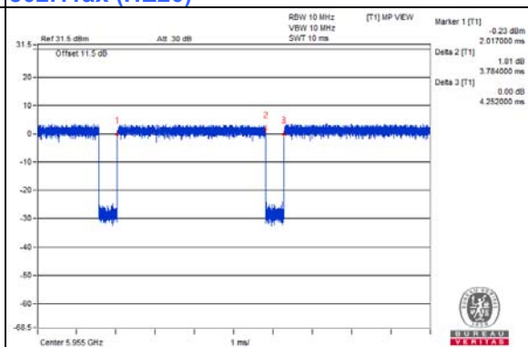
802.11ax (HE80)
