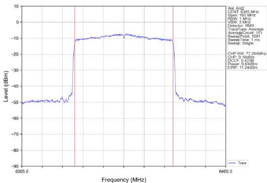
802.11ax(HEW80)_HCH_6385MHz_SU_Ant2_NTNV
