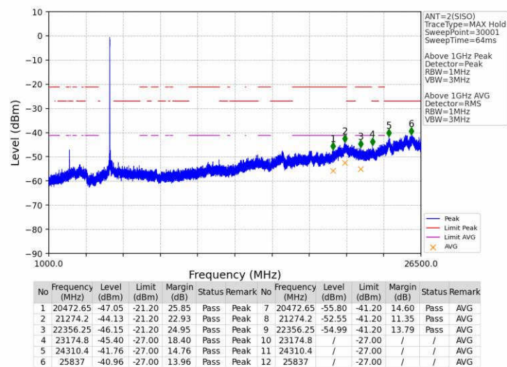
802.11a_LCH_5180MHz_Ant2_NTNV
