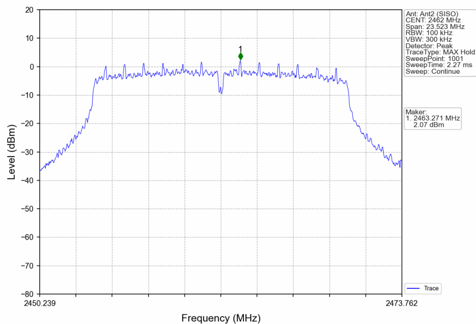
802.11g HCH 2462MHz Ant2 (SISO) NTVN
