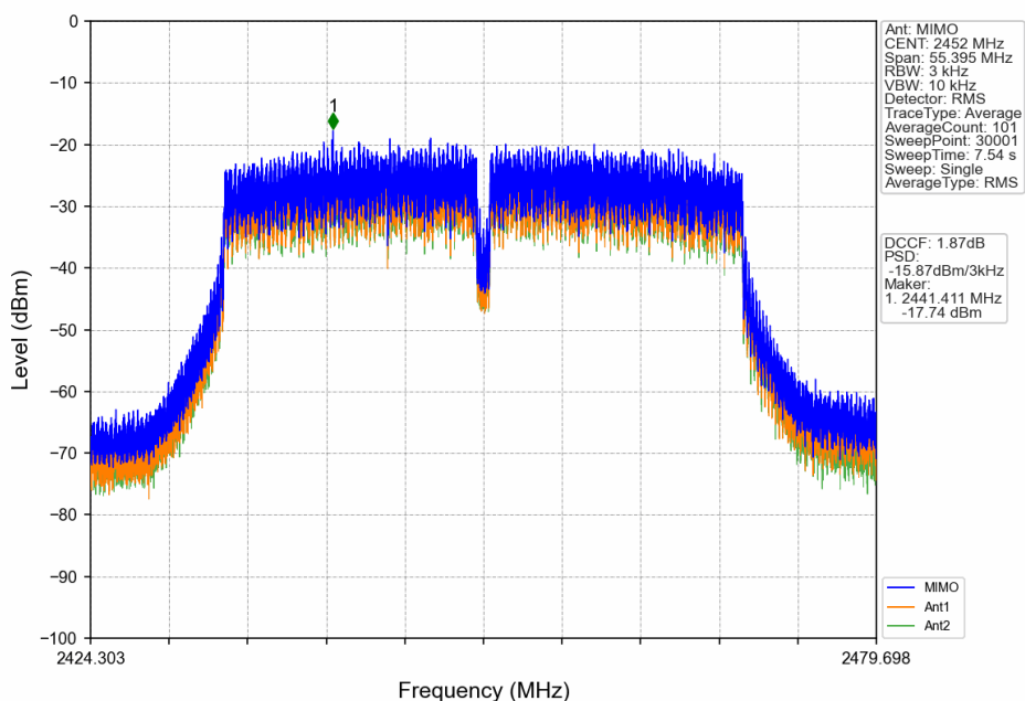
802.11n(HT40) HCH 2452MHz MIMO NTN
