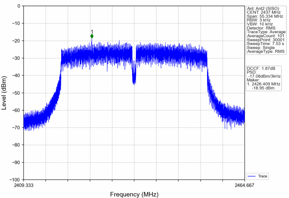
802.11n(HT40) MCH 2437MHz Ant2 (SISO) NTN
