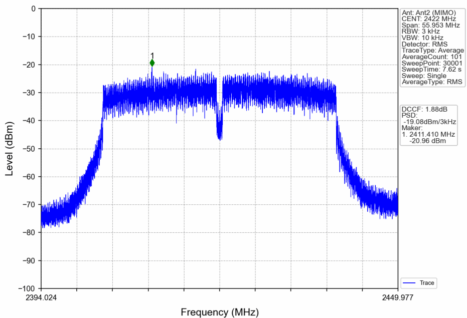
802.11n(HT40) LCH 2422MHz MIMO NTNV
