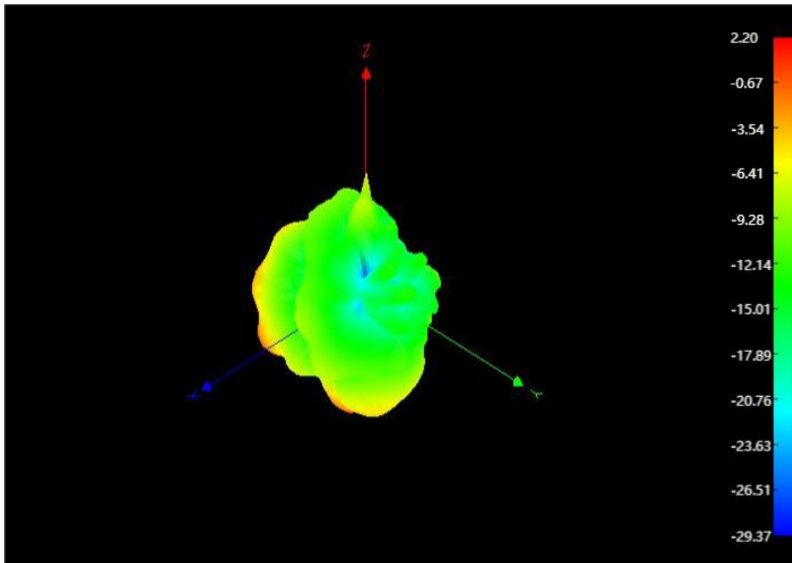
2400MHz 3D
