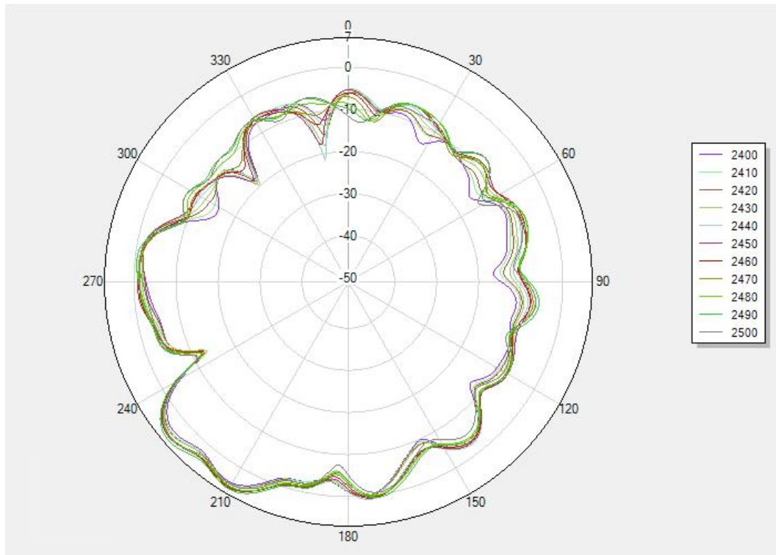
2400MHz 3D
