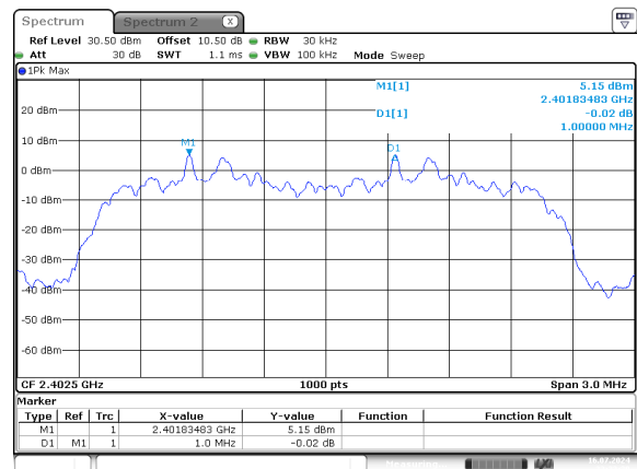
\pi/4 -DQPSK_Low
