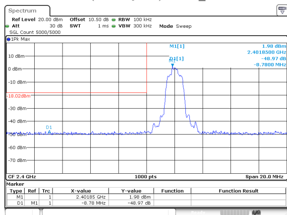
EDR( \pi/4 -DQPSK) 2DH1_Low
