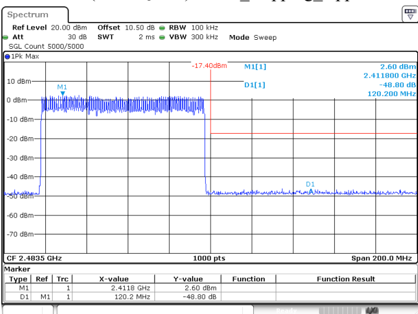
EDR( \pi/4 -DQPSK) 2DH1_Hopping_Upper
