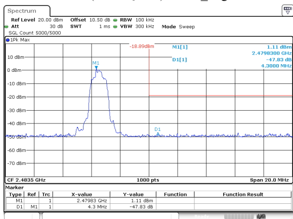
EDR( \pi/4 -DQPSK) 2DH1_High
