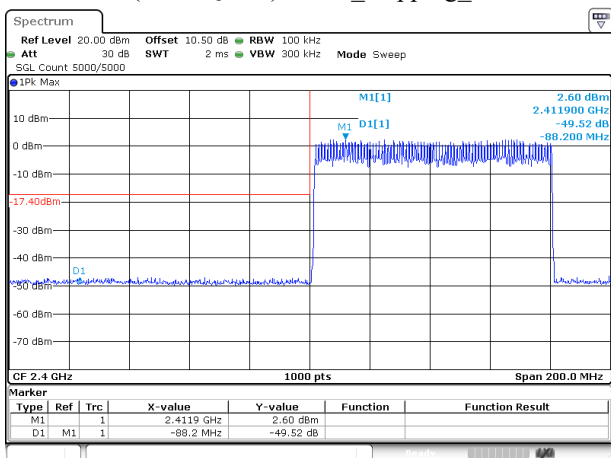
EDR( \pi/4 -DQPSK) 2DH1_Hopping_Lower
