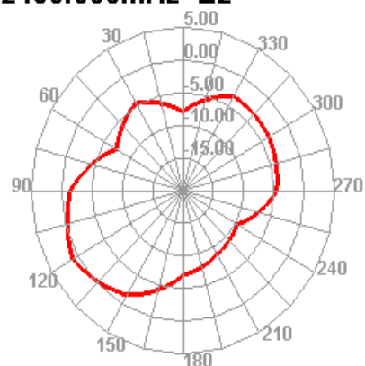
2450.000MHz E2
