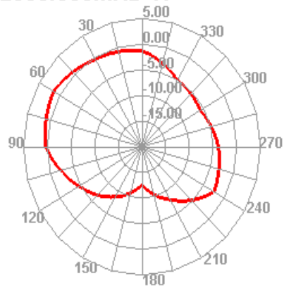
2500.000MHz H
