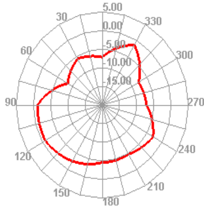
5150.000MHz H
