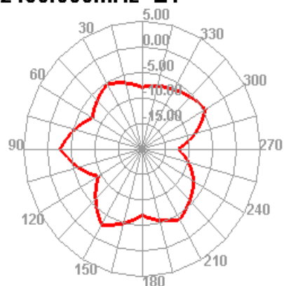
2450.000MHz E1
