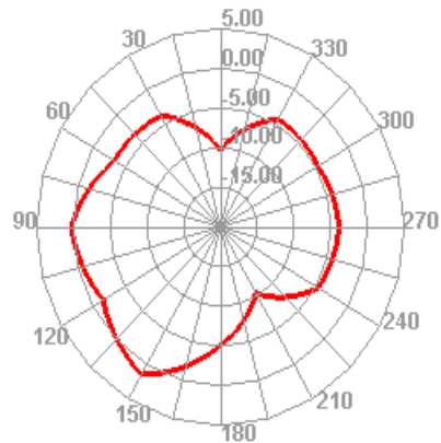
2500.000MHz E2
