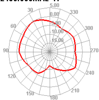
2450.000MHz H
