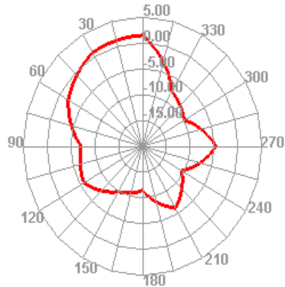
5150.000MHz E1
