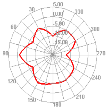
2500.000MHz E1
