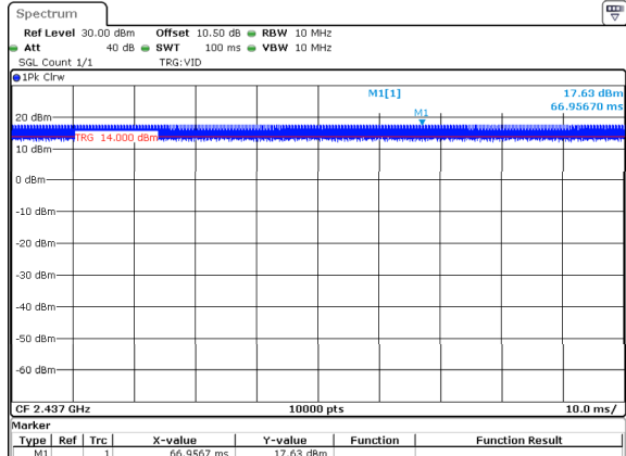
802.11g_2437MHz
