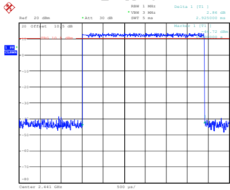
3DH5_Hopping 2.925ms
