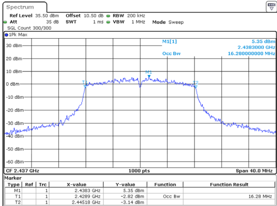
802.11g_2437MHz 16.280MHz
