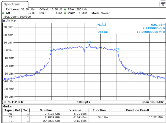
802.11g_2412MHz 16.320MHz
