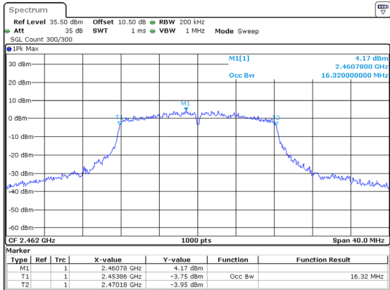
802.11g_2462MHz 16.320MHz
