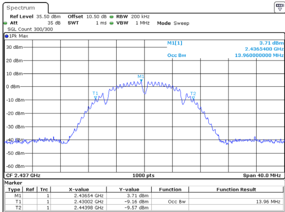
802.11b_2437MHz 13.960MHz
