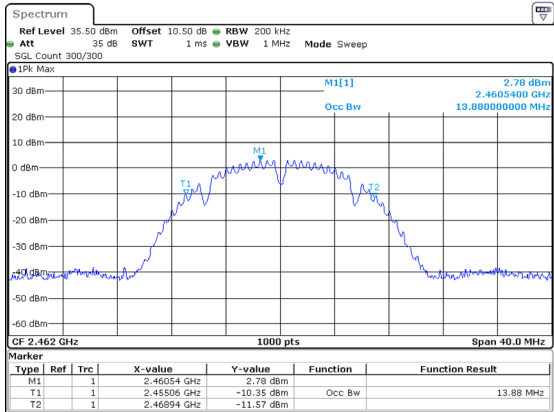
802.11b_2462MHz 13.880MHz
