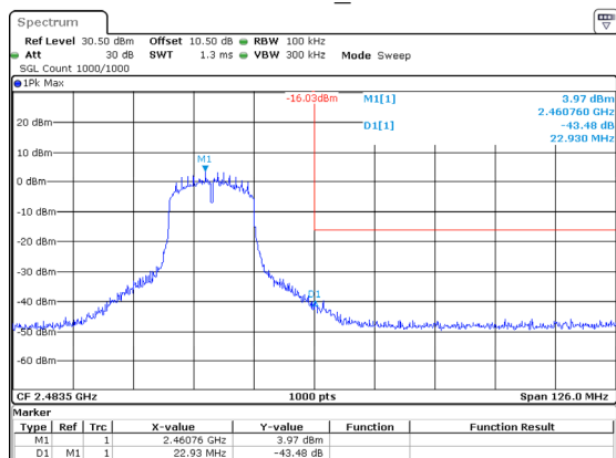
802.11n-HT20_2462MHz
