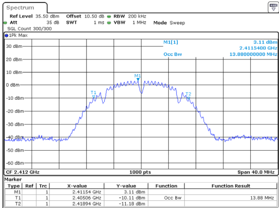
802.11b_2412MHz 13.880MHz
