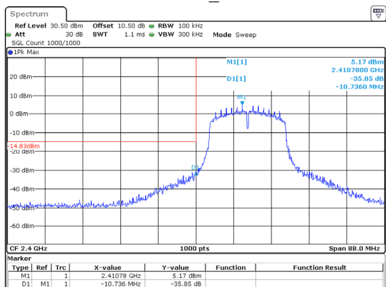
802.11n-HT20_2412MHz
