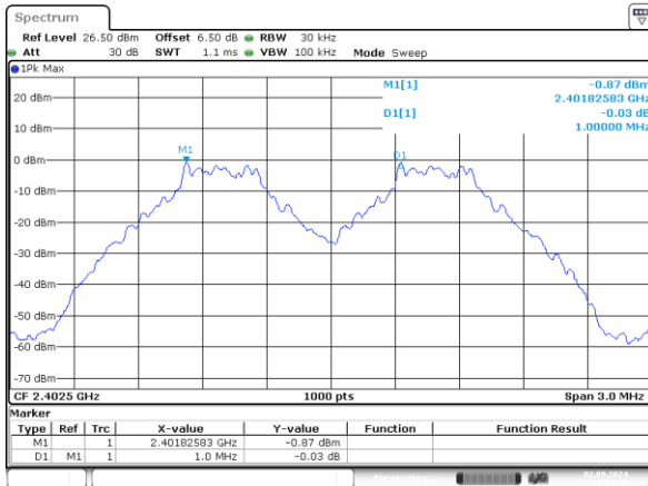
GFSK_Low 1MHz
