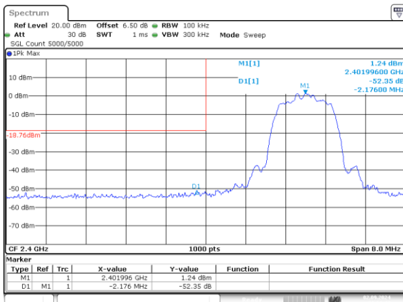
\pi/4 -DQPSK_Low 52.35dB
