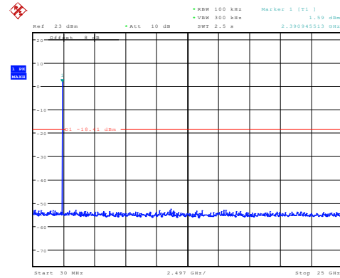
\pi/4 -DQPSK_Low
