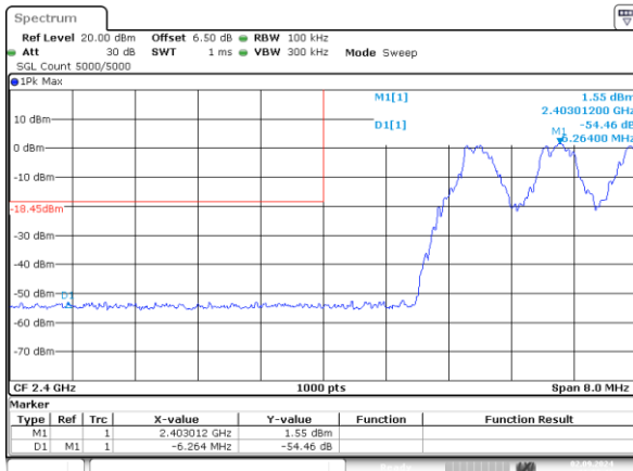
GFSK_Hopping_Lower 54.46dB
