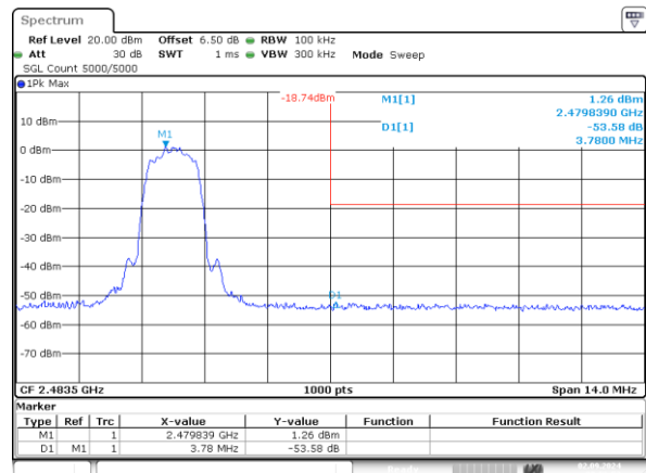
\pi/4 -DQPSK_High 53.58dB
