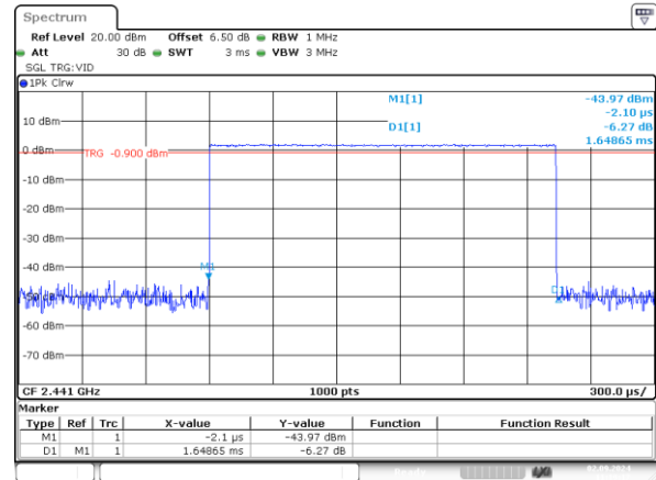
GFSK_Hopping_DH3 1.649ms
